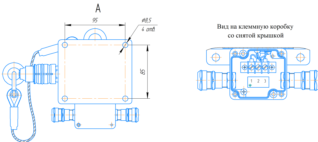
Рисунок 1. Габаритный чертеж
